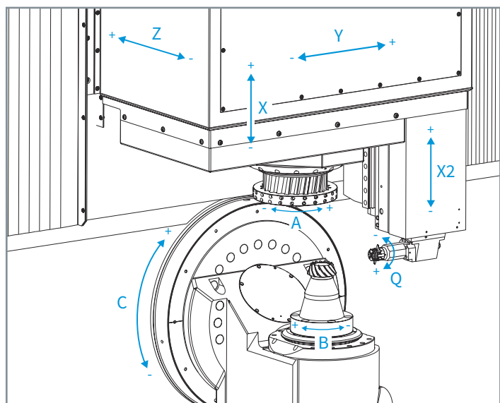
Oerlikon（奥利康）C 30 锥齿轮切齿机的轴线示意图
