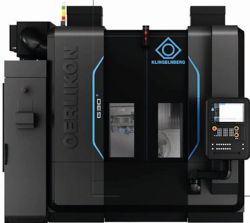
Oerlikon Kegelradschleifmaschine G 30 mit zahlreichen Ausstattungsdetails
