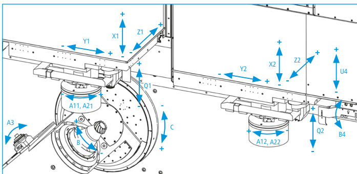
Achsanordnung einer Oerlikon Kegelrad-Schleifmaschine G 35
