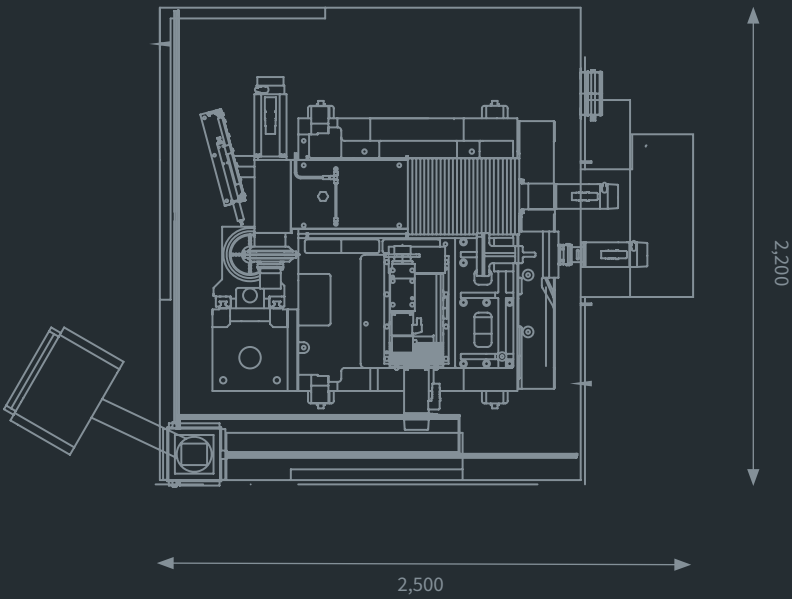
HELIX 400: 俯视图
