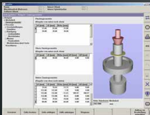
Grafische Eingabe der Zusatzgeometrie zur Kollisionskontrolle
