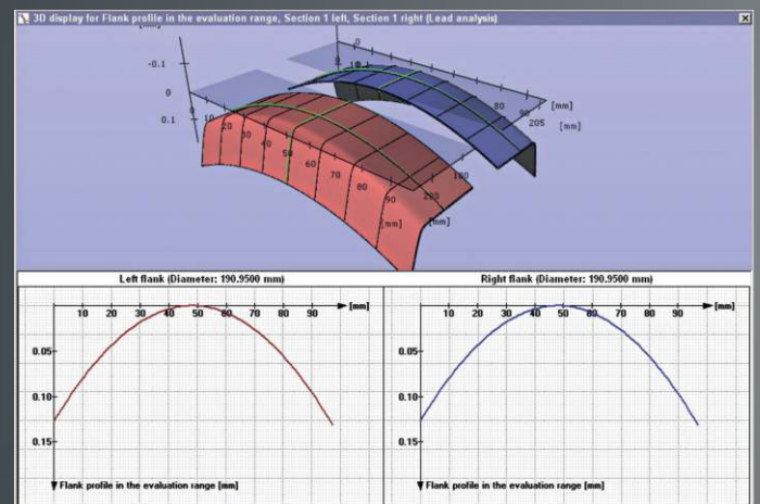
齿面形状的3D模拟分析
