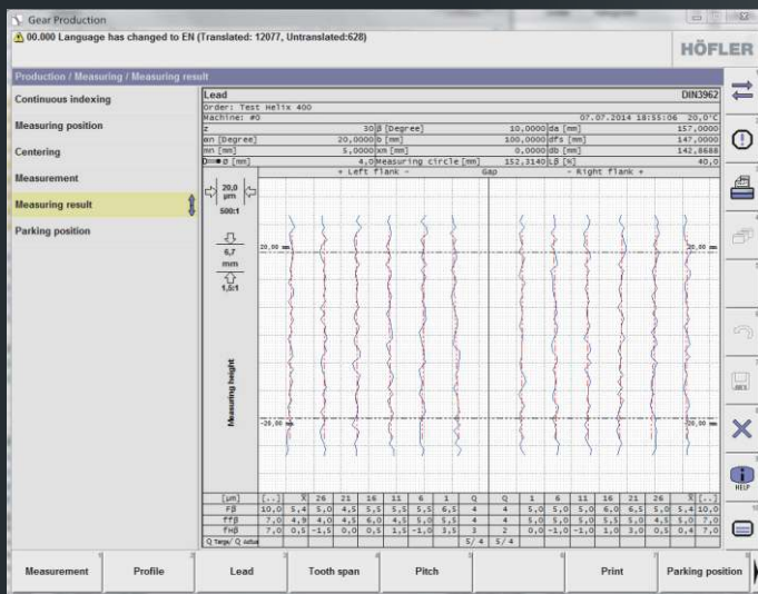
在线测量
