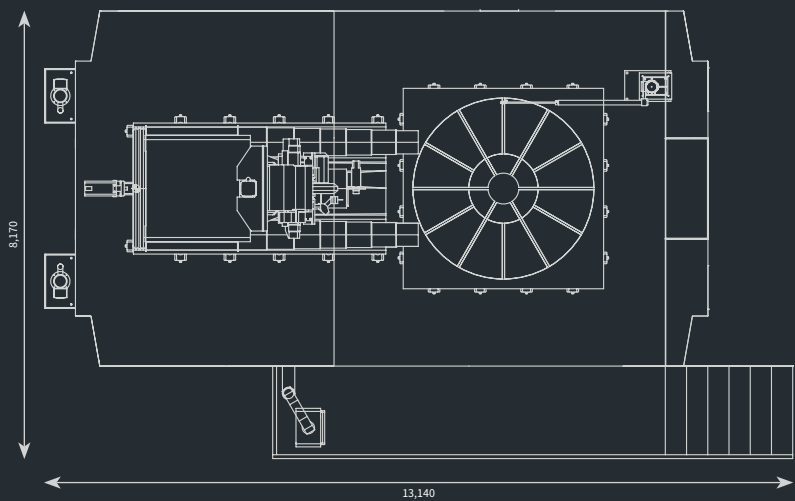
RAPID 6000：俯视图
