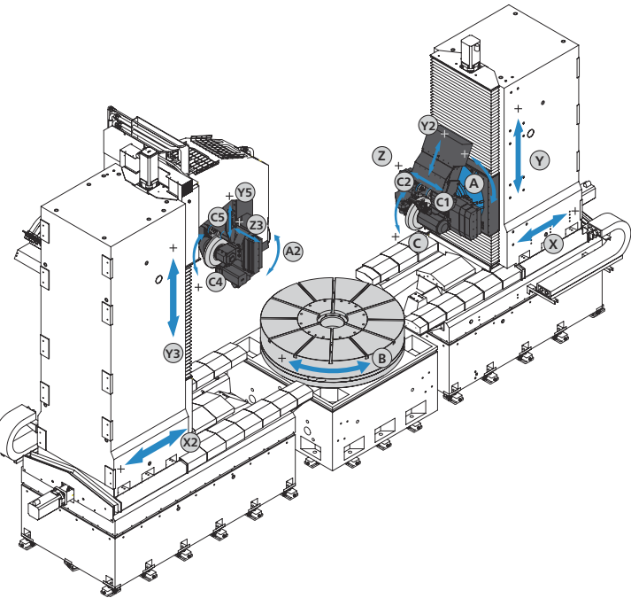
以RAPID 4000 AI型磨齿机为例的轴线示意图
