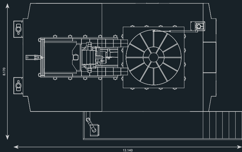
RAPID 6000: Draufsicht
