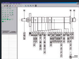
Maß, Form und Lage (Welle) – Übersichtliche Bedienoberfläche mit Darstellung der Messparameter und Messblätter
